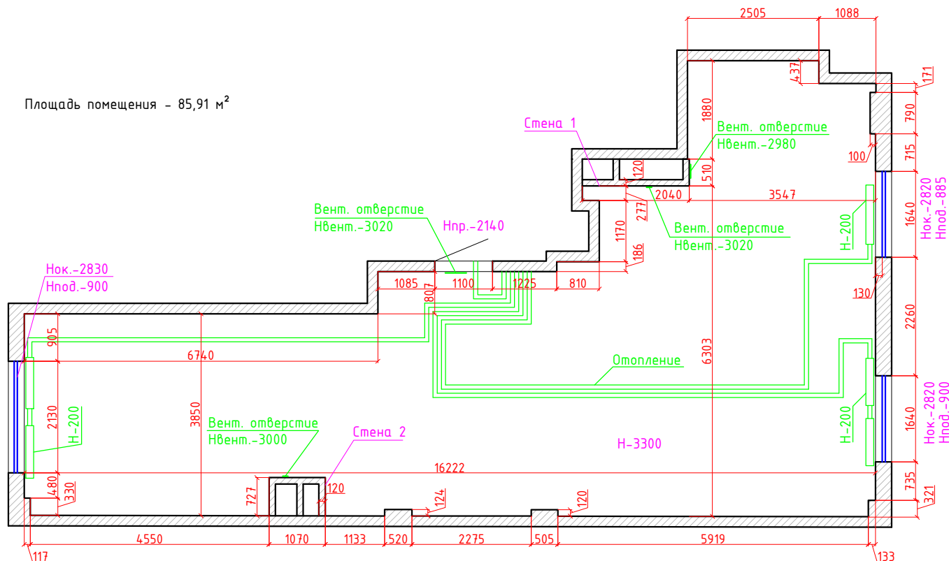
Стена 1 Схема расположения ревизионных отверстий М 1:50
